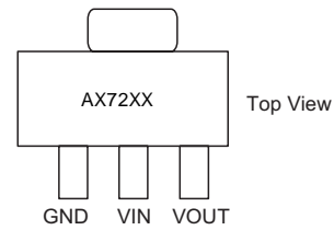
SOT89
